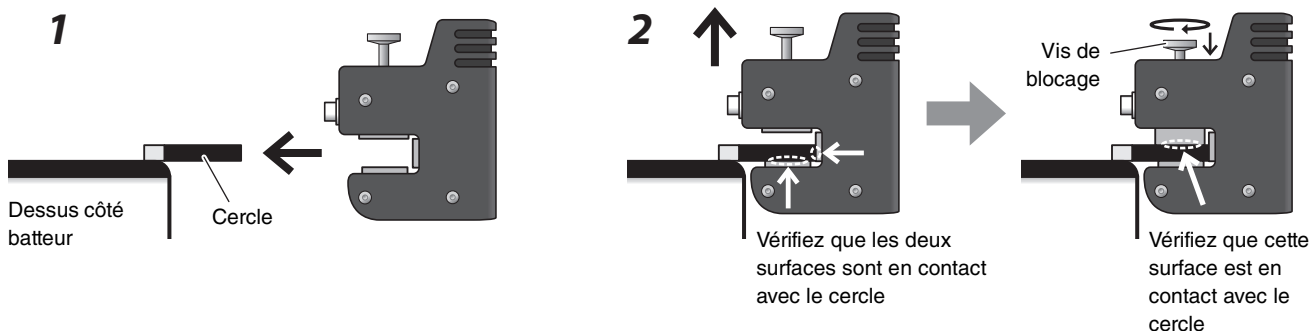
Vue latérale
