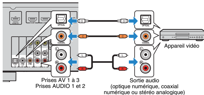
L'unité (arrière)
