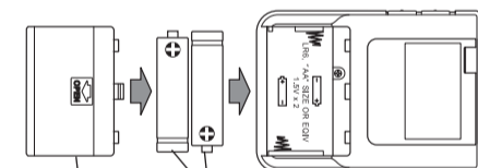
Couvercle du logement des piles Deux piles AA alcalines ou nickel-métal hydrure
